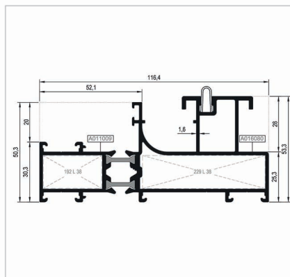
1083 AT116 F 16 2,406 Kg/mt
