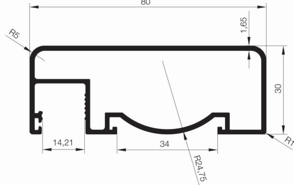
1007 A80 T 01 1,110 Kg/mt
