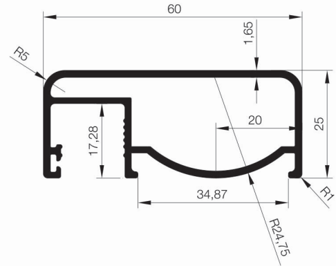
1011 A60 T 01 0.830 Kg/mt
