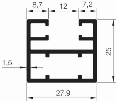
1002 AS38 T 08 0.537 Kg/mt
