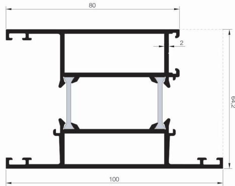
1072 T64 K 01 2,337 Kg/mt
