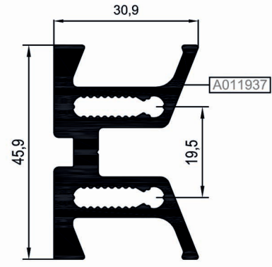
1096 R50 C 24 1,363 Kg/mt
