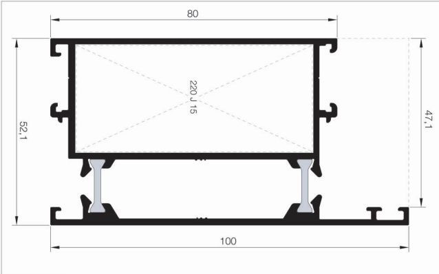
1077 T116 F 03 1,935 Kg/mt
