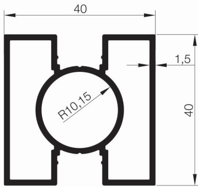
1018 A400 D 02 0,960 Kg/mt
