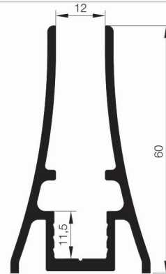
1013 A40 C 01 1.007 Kg/mt
