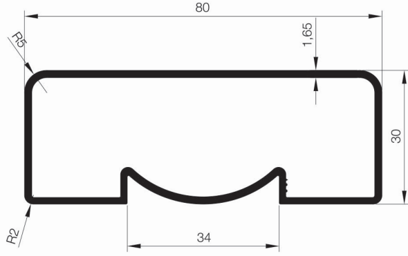
1008 A80 T 02 0,985 Kg/mt
