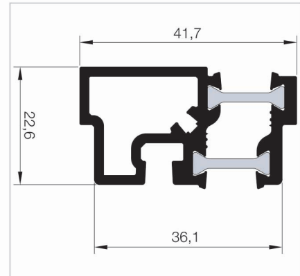
1081 T116 A 04 0,867 Kg/mt
