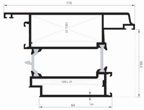
1070 T64 V 06 2,827 Kg/mt
