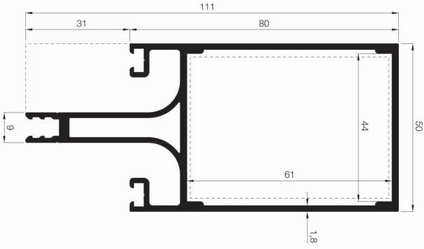
1085 R50 M 01 1,956 Kg/mt
