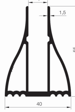
1001 AS38 T05 1,011 Kg/mt
