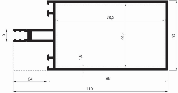
1088 R50 T 04 1,640 Kg/mt
