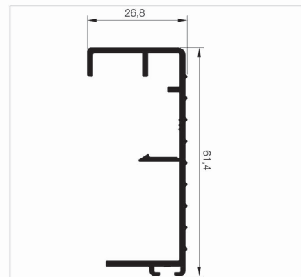
1084 T116 A 10 0,553 Kg/mt
