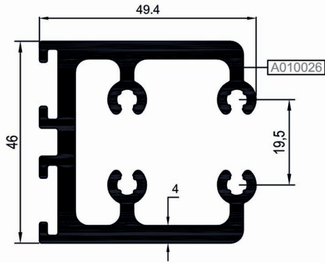
1095 R50 C 06 2,033 Kg/mt
