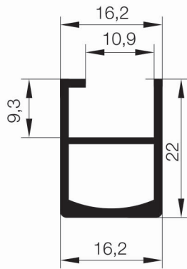
1012 A40 C 03 0.270 Kg/mt
