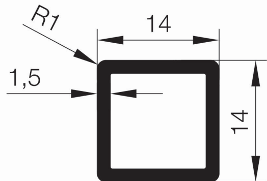
1015 A40 A 01 0.201 Kg/mt
