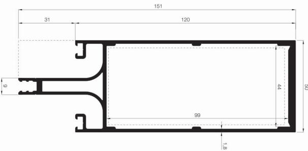
1087 R50 M 03 2,608 Kg/mt
