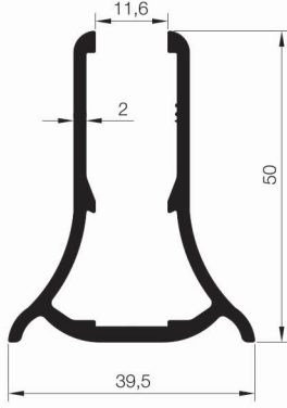
1000 AS38 T 04 0,834 Kg/mt
