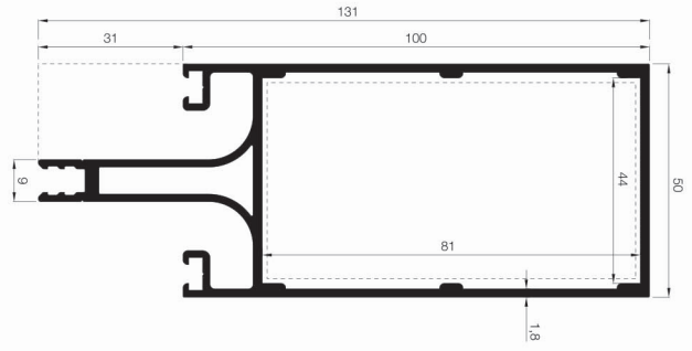
1086 R50 M 02 2,159 Kg/mt
